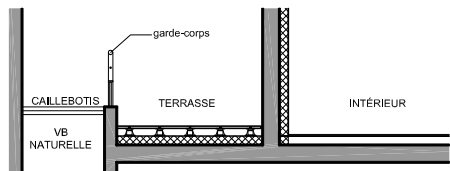
COUPE AA SUR LA TERRASSE
