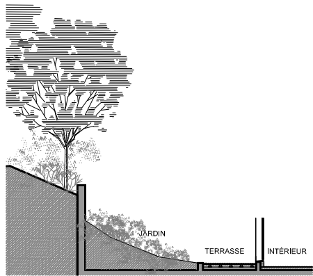
COUPE DE PRINCIPLE SUR LE JARDIN
