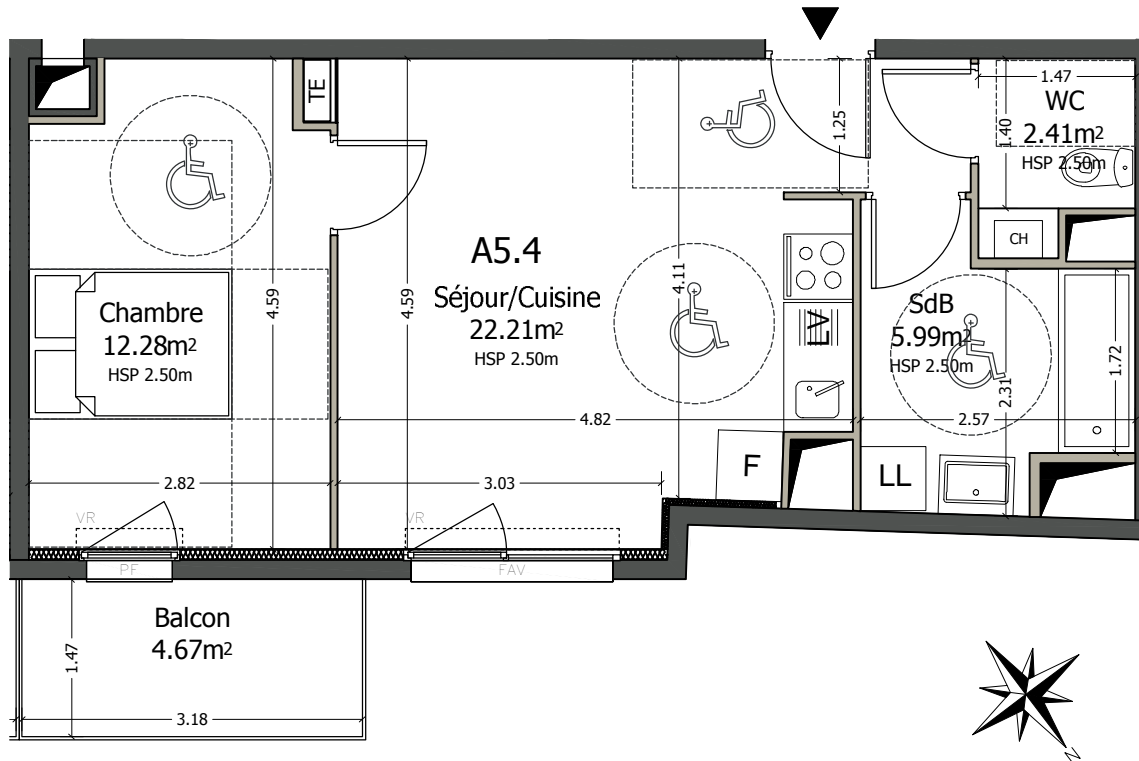
PLAN DU LOGEMENT
